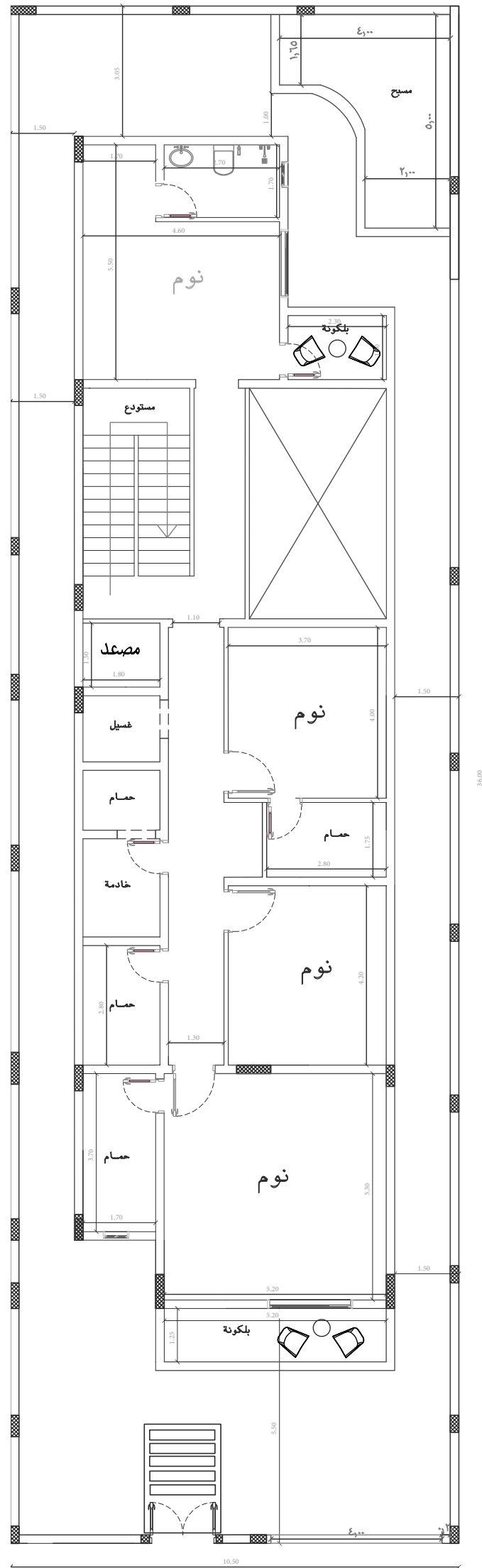
مخطط الدور الأول
