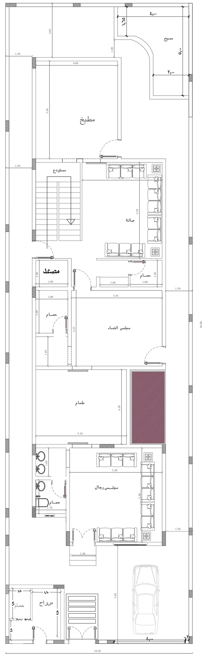
مخطط الدور الأرضي
